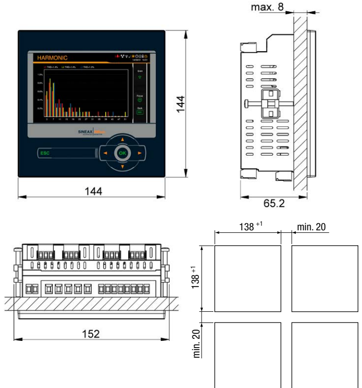
Schalttafelauausschnitt
