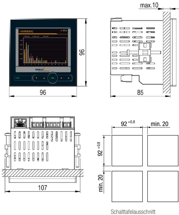
Schalttafelauausschnitt
